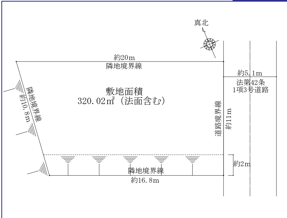
概略地形図
